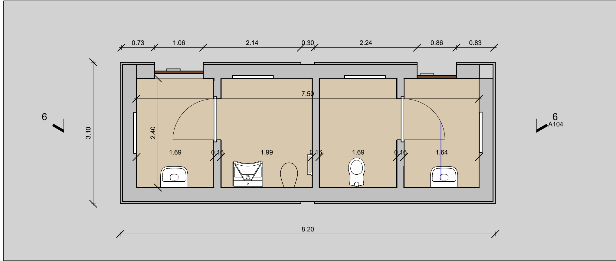
0 - Piano Terra_STATO DI FATTO a 1:50
