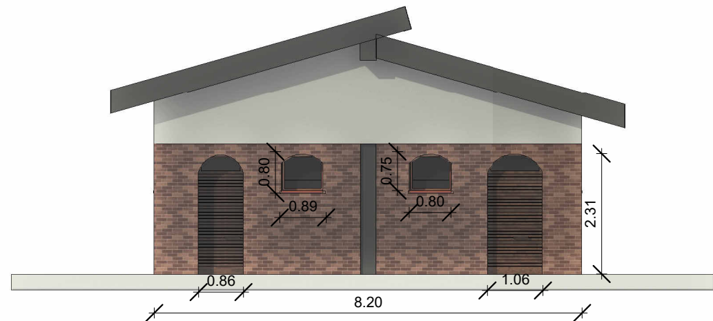
Nord Scal a 1:100
