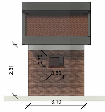
Ovest Scal a 1:100
