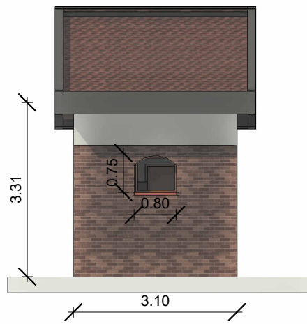
Est Scal a 1:100
